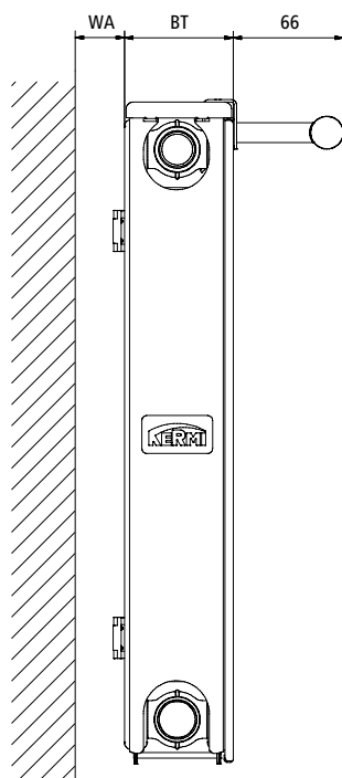
Стальные панельные радиаторы Plan / Line
