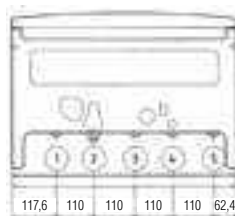
ВИД СНИЗУ
