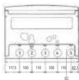
ВИД СНИЗУ
